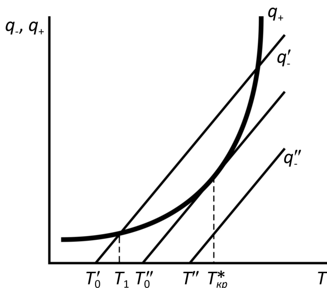
Рисунок 5 – Диаграмма Семёнова
